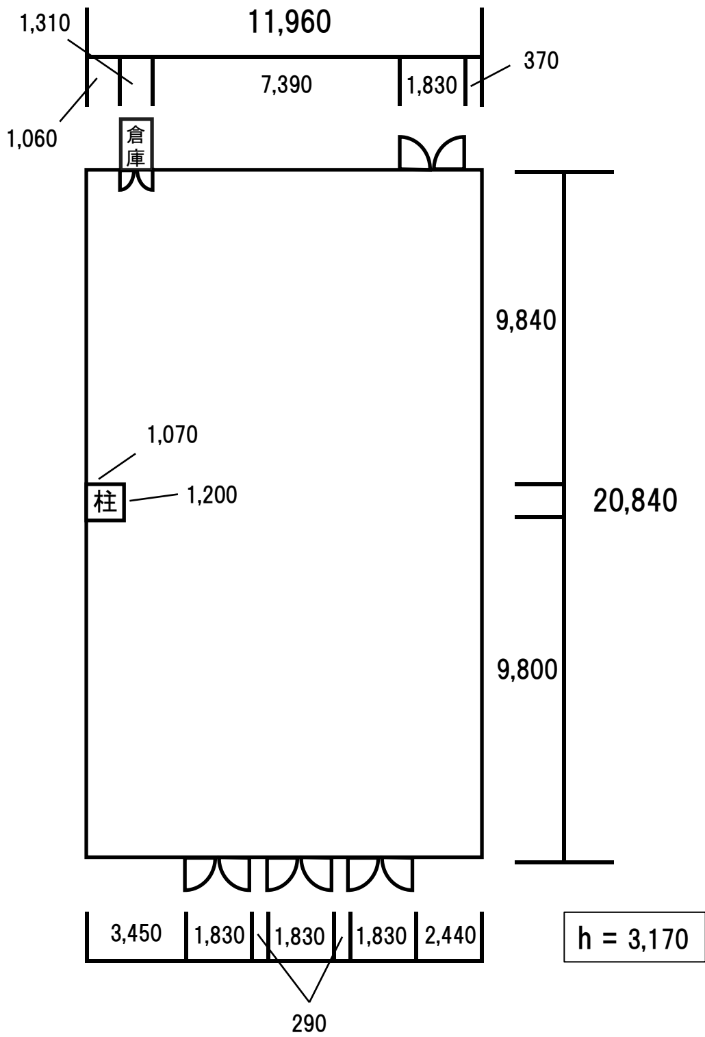
大船渡市魚市場3階多目的ホール簡易図面
